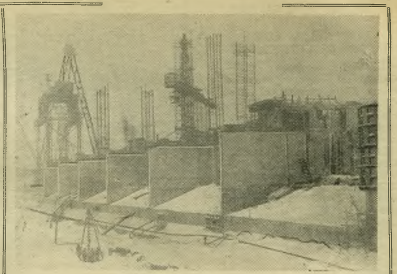
На Волге близ города Горького сооружается крупная гидроэлектростанция. Строители досрочно выполнили план земляных работ в котлованах здания ГЭС, водосливной плотины и шлюзов. Полным темпом идут строительные-монтажные работы.
