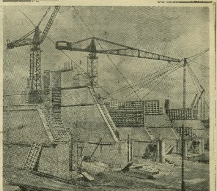
Молдавская ССР. Недалеко от районного центра Дубоссары строится первая на реке Днестр гидроэлектростанция. Сооружается водосливная плотина, здание электростанции, монтируются турбины. Коллектив строителей уложил уже 65 процентов бетона и выполнил 85 процентов земляных работ. С вводом в эксплуатацию Дубоссарская ГЭС будет снабжать электроэнергией прилегающие промышленные районы и сельское хозяйство.
