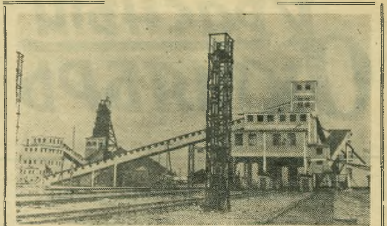
Сталинская область. Шахта № 1 «Родинская» треста «Красноармейскуголь» вступила в строй в этом году. Все процессы добычи и доставки угля здесь полностью механизированы. Горняки новой шахты на месяц раньше срока выполнили семимесячное задание.
