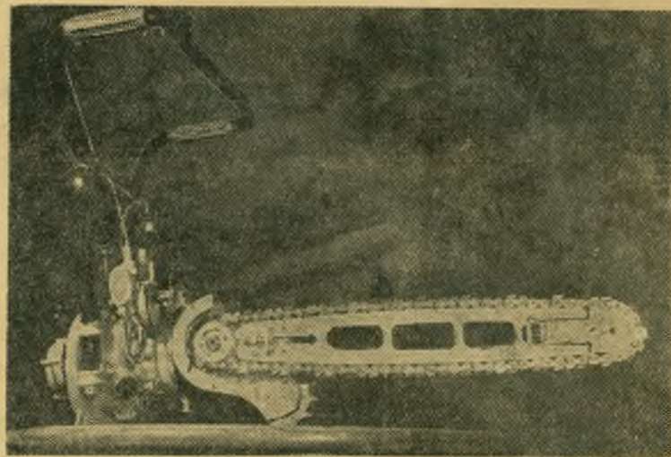
Советские ученые совместно с производственниками разработали новую конструкцию бензиномоторной цепной пилы, предназначенной для валки и раскряжевки деревьев, а также вспомогательных работ по прорубке и расчистке трасс, строительству деревянных сооружений и т. д. Вес облегченной пилы новой конструкции снижен до 10,5 килограмма, мощность одноцилиндрового двухтактного бензинового двигателя осталась прежней—3,2 лошадиных силы.
