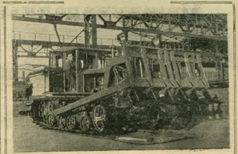
Украинская ССР. В экспериментальном цехе Николаевского завода «Дормашина» закончено изготовление опытных образцов корчевателей на тракторах «ДТ-54» и «ДТ-55», предназначенных для корчевки пней и кустарников при освоении целинных и залежных земель.
