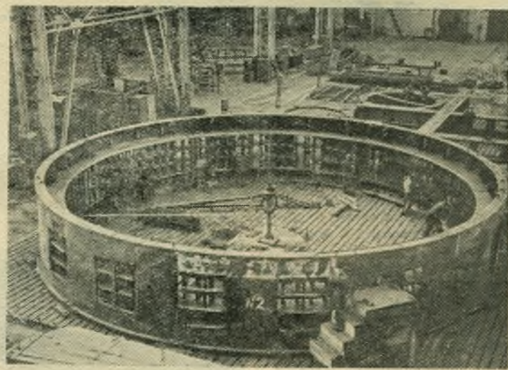
Харьков. На заводе тепловозного электрооборудования изготавливается мощный гидротурбинный генератор для Каховской ГЭС. НА СНИМКЕ: сборка статора гидротурбинного генератора. Фото М. Начинкина. (Фотохроника ТАСС).
