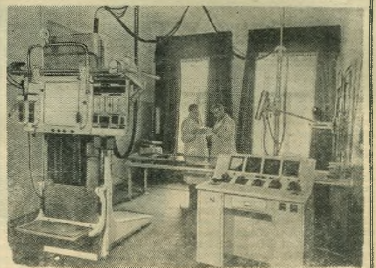
Московский завод «Мосрентген» создал для исследования больных универсальную рентгеновскую установку «РУМ-5». В ней применены более совершенные рентгеновские трубки. Управление автоматизировано.
