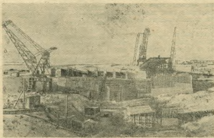
На строительстве Новосибирской гидроэлектростанции. НА СНИМКЕ: общий вид работ в котловане под зданием ГЭС. Фото В. Лецинского. (Фотохроника ТАСС).
