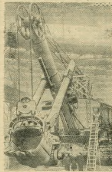
Свердловск. Коллектив Уралмашзавода изготовил скальный экскаватор. В час он может вынуть более 2.000 тонн руды. Емкость ковша машины 6 кубометров. За две с половиной минуты им загружается 60-тонный железнодорожный вагон. НА СНИМКЕ: скальный шестикубовый экскаватор. Фото А. Грахова.
