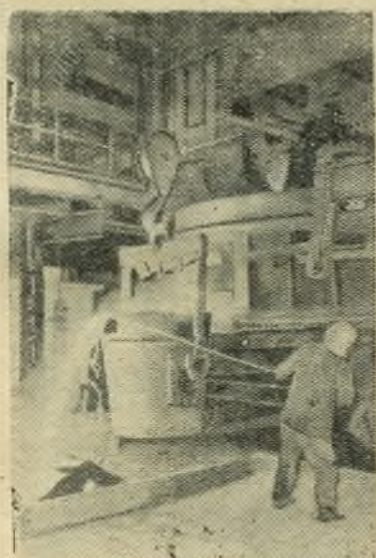
Грузинская ССР. На Зестафонском заводе ферросплавов недавно пущена первая очередь цеха рафинированного ферромарганца. В цехе механизированы и автоматизированы производственные процессы. Здесь установлены вращающиеся и наклоняющиеся ферросплавные печи. Дозировка шихтовых материалов и подача шихты в печи полностью механизированы.
