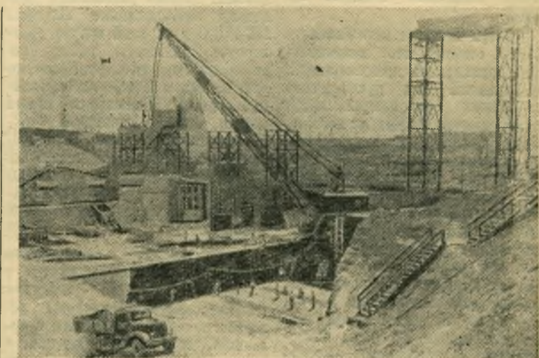
Таджикская ССР. Строительство Кайрак-Кумской гидроэлектростанции на реке Сыр-Дарье.
