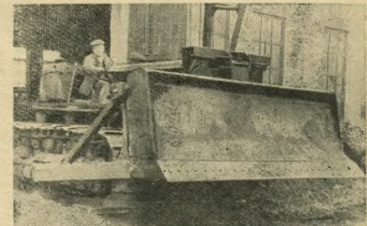
Ремонтно-механический завод объединения «Куйбышевнефть» изготовляет навесное оборудование для бульдозеров, при помощи которого производится рытье силосных траншей в колхозах и совхозах. НА СНИМКЕ: тракторист тов. Орлов выезжает из ворот цеха ремонтно-механического завода на испытание навесного бульдозерного оборудования. Фото В. Владимиров.
