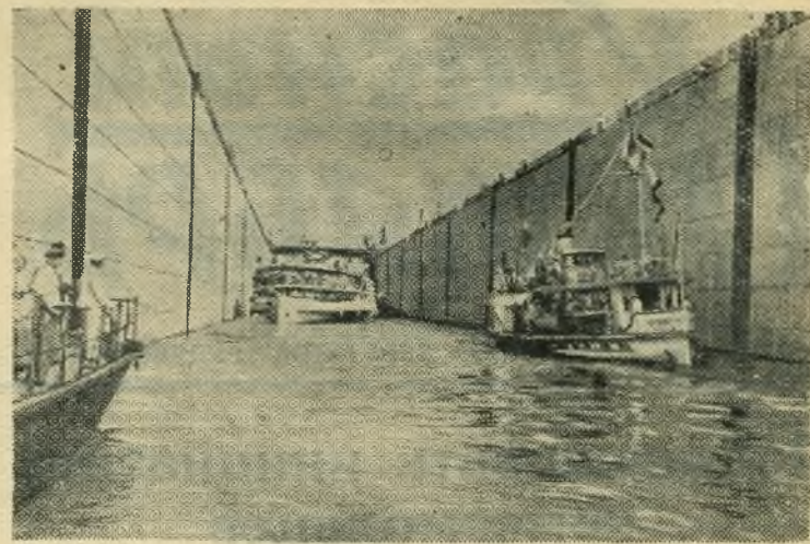
Недавно на строительстве Куйбышевской гидроэлектростанции состоялся пуск нижних судоводных шлюзов. НА СНИМКЕ: шлюзование первых судов. Фото А. Батанова. (Фотохроника ТАСС).
