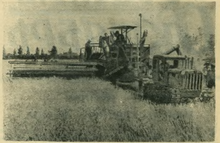
В июле этого года на Пекинском заводе сельскохозяйственного машиностроения закончено изготовление первого китайского комбайна. Машина была сконструирована по типу советского комбайна «Сталинец-6». В создании комбайна оказали помощь советские инженеры.
