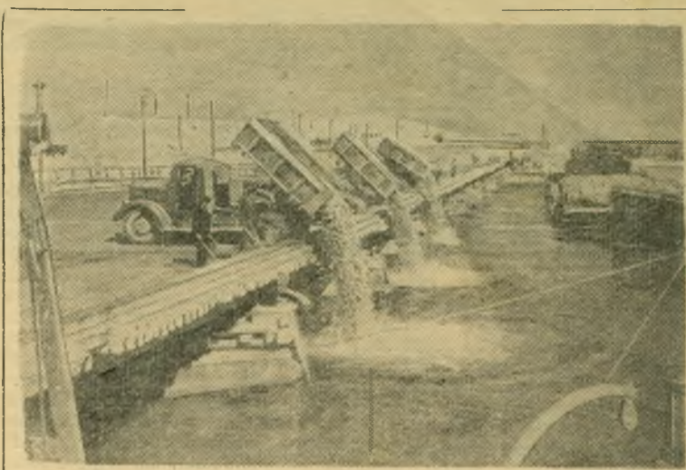
На строительстве Горьковской гидроэлектростанции. НА СНИМКЕ: момент перекрытия русла Волги. Фото П. Вознесенского. (Фотохроника ТАСС).
