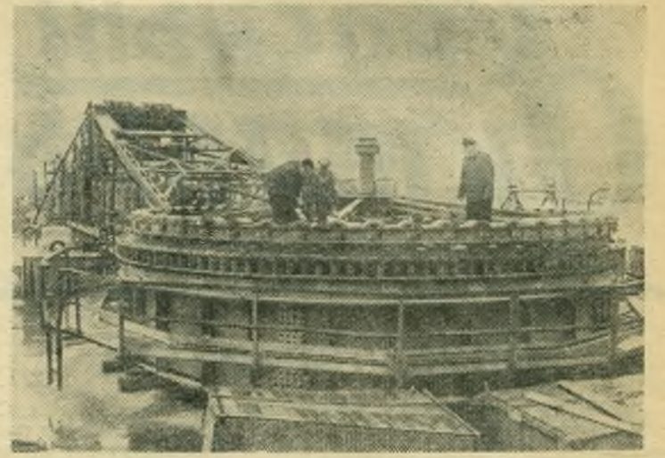
Ленинград. Судоремонтный завод треста «Балттехфлот» спустил на воду пловучий самоходный кран грузоподъемностью в 50 тонн. Длина его 40 метров, ширина—20 метров, общий вес — около 1.500 тонн. Сейчас слесари-монтажники приступили к сборке металлоконструкций и механизмов крана. Ввод его в действие обеспечит механизацию трудоемких работ в гидротехническом строительстве и на ремонте судов технического флота.
