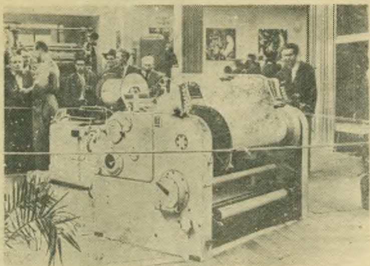
Чехословацкая Республика. Бесшумный ткацкий станок, изобретенный чехословацким инженером. Роль челнока в станке исполняет капля воды. Под давлением в пять атмосфер она вылетает из форсунки и увлекает за собой нить, укладывая в течение часа 20 тысяч нитей.
