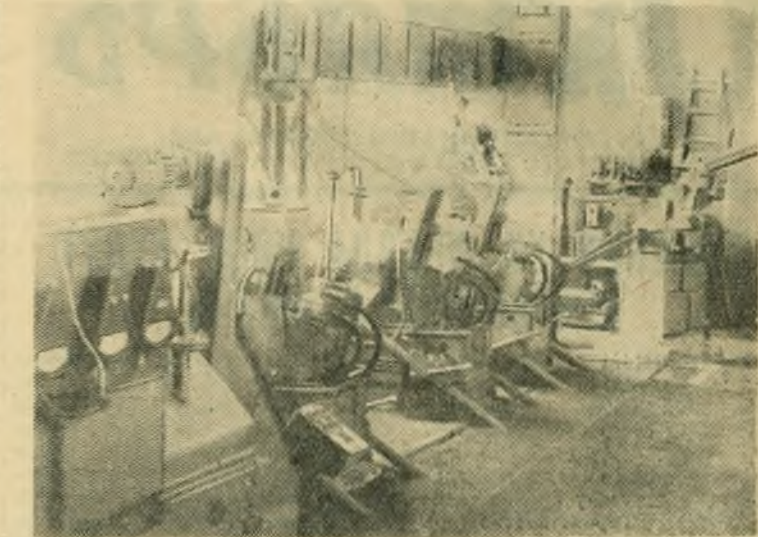
На комбайновом заводе продолжается автоматизация производственных процессов. В цехе № 16 действует автоматическая линия по изготовлению гаек. Ее производительность — 26 тысяч гаек в смену. В текущем году будет создана механизированная линия по производству балансирующих пружин для силосоуборочных комбайнов. НА СНИМКЕ: автоматическая линия по изготовлению гаек. Фото В. Грачева.
