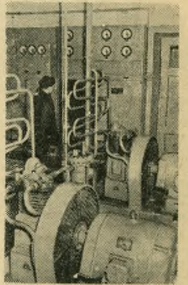
Московская область. Под Ногинском построена подстанция для приема электроэнергии с Куйбышевской ГЭС. Напряжение 400.000 вольт здесь будет понижаться до 220.000 и 110.000 вольт.
