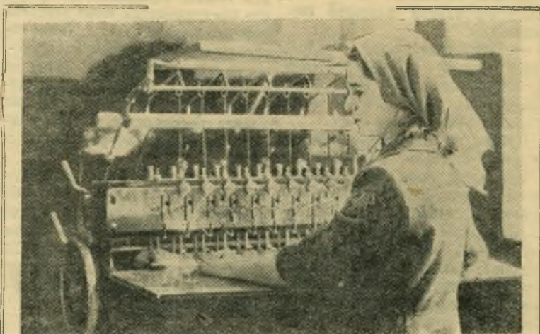
Новая техника на предприятиях города. Недавно швейная фабрика № 14 пополнилась новой 12-игольной стегальной машиной. Выпущенной Киевским экспериментальным механическим заводом. Этой машиной производится стеганая ватина к зимним пальто.
