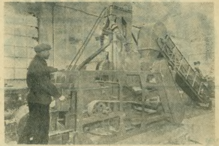
Харьков. Группа инженеров и механиков областного мельничного треста сконструировала и изготовила малогабаритную передвижную фуражную мельницу для переработки кукурузы. Ее производительность — до 20 тонн в сутки. Испытания дали положительные результаты.
