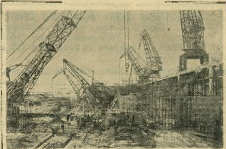
Строителям Новосибирской гидроэлектростанции в нынешнем году предстоит уложить 290 тысяч кубометров бетона, произвести намыв в русловую и левобережную части плотины большого количества грунта, смонтировать 7600 тонн металлоконструкций. На всех участках стройки развернулось соревнование за досрочное выполнение плана первого года шестой пятилетки.
