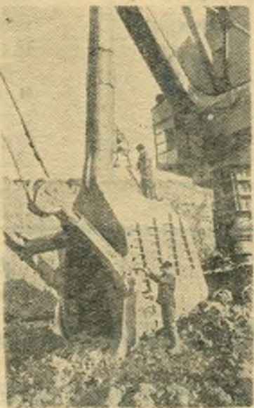
Свердловская область. Трест «Вахрушевуголь» ведет открытую добычу угля. На угольных разрезах и вскрышных работах применяются мощные машины. План первых двух месяцев коллектив перевыполнил. НА СНИМКЕ: подготовка к работе электрической гусеничной лопаты «ЭГЛ-15» в бригаде мастера И. Орлова. Бригада вынимает до 5.000 кубометров породы в смену при норме 3.300 кубометров. Фото Л. Великанова. (Фотохроника ТАСС).
