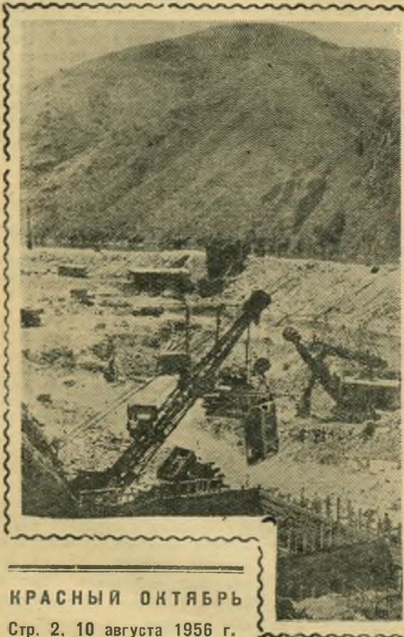
Восточно-Казахстанская область. Строители Вухтарминской ГЭС наращивают темпы укладки бетона в водосливную часть плотины гидроузла. Завершено бетонирование первых двух блоков. Начата укладка бетона в третий блок. По объему он значительно больше предыдущих, вместе взятых. НА СНИМКЕ: укладка бетона в третий блок. Фото Г. Емельянова. (Фотохроника ТАСС).
