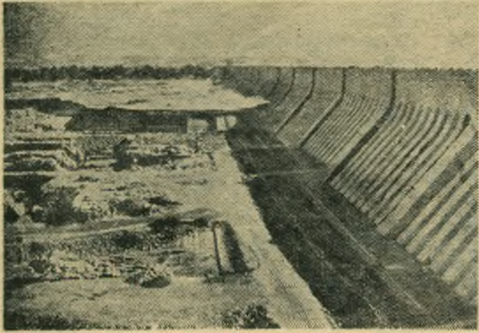
Египет. Часть строящейся Асуанской плотины. Фото агентства Кейстон.
