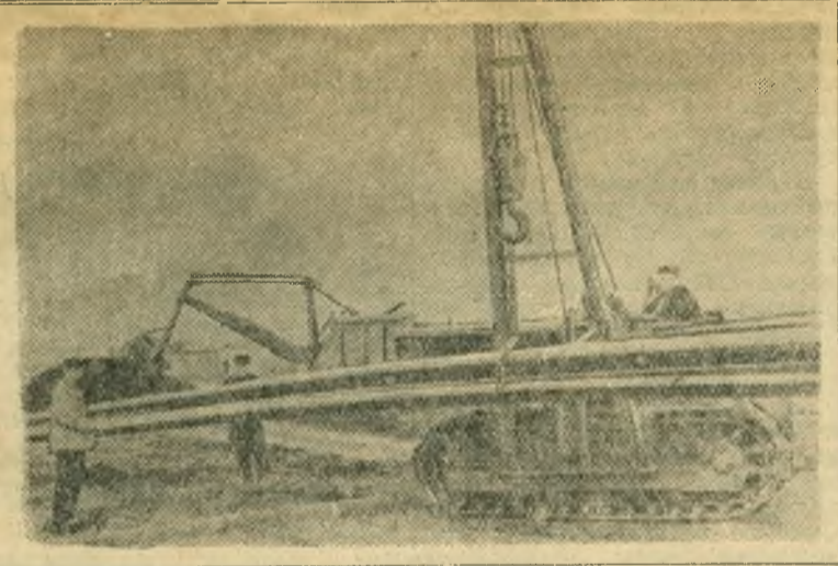
На строительстве поселка «Образцовский» ведутся работы по сооружению водопровода. НА СНИМКЕ: тракторист Г. Рафинов развозит водопроводные трубы. Фото Ф. Шнарбаненно.
