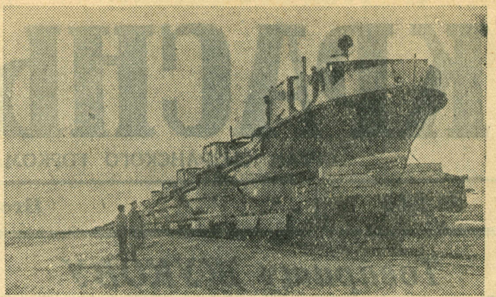
Астраханская область. Завод «Красные баррикады» Министерства нефтяной промышленности СССР освоил выпуск речных судов-буксировщиков с двигателями в 150 лошадиных сил. На реках Обь и Иртыш новые суда будут использоваться для буксировки барж с оборудованием геофизических и геологических партий.
