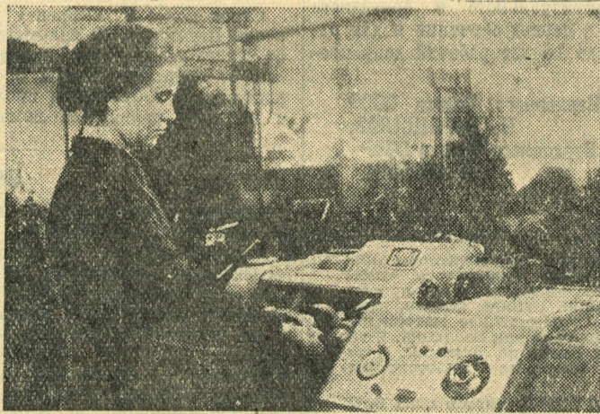
На комбайновый завод поступает много самой совершенной техники. Недавно в цеху № 16 был установлен новый резьбо-накатный станок, привезенный из Чехословакии. С помощью этого станка полуавтоматом цех намного увеличил выпуск болтов и другого крепежного материала и тем самым полностью обеспечил им сборщиков. На снимке: резьбонакатчица Галина Анисимова за работой на новом станке. Фото П. Корчагина.
