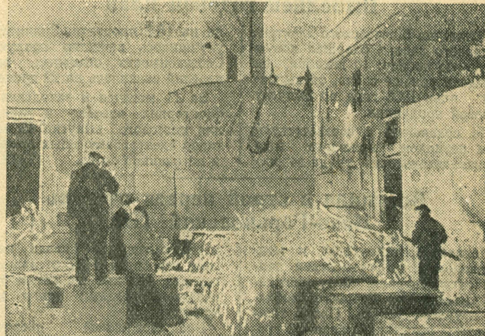
Ленинград. Коллектив Ижорского завода изготовил около двух тысяч листов для обшивки и внутренних переборок корпуса будущего атомного ледокола. Они уже отправлены на верфь. Сейчас здесь делают плиты для ограждения атомного реактора и другие конструкции.
